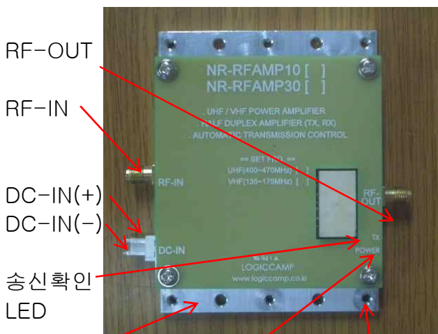
기본 알루미늄 방열판 전원 LED 고정용 홀(Hole) 팬(FAN) 케이스 고정용 육각보스
